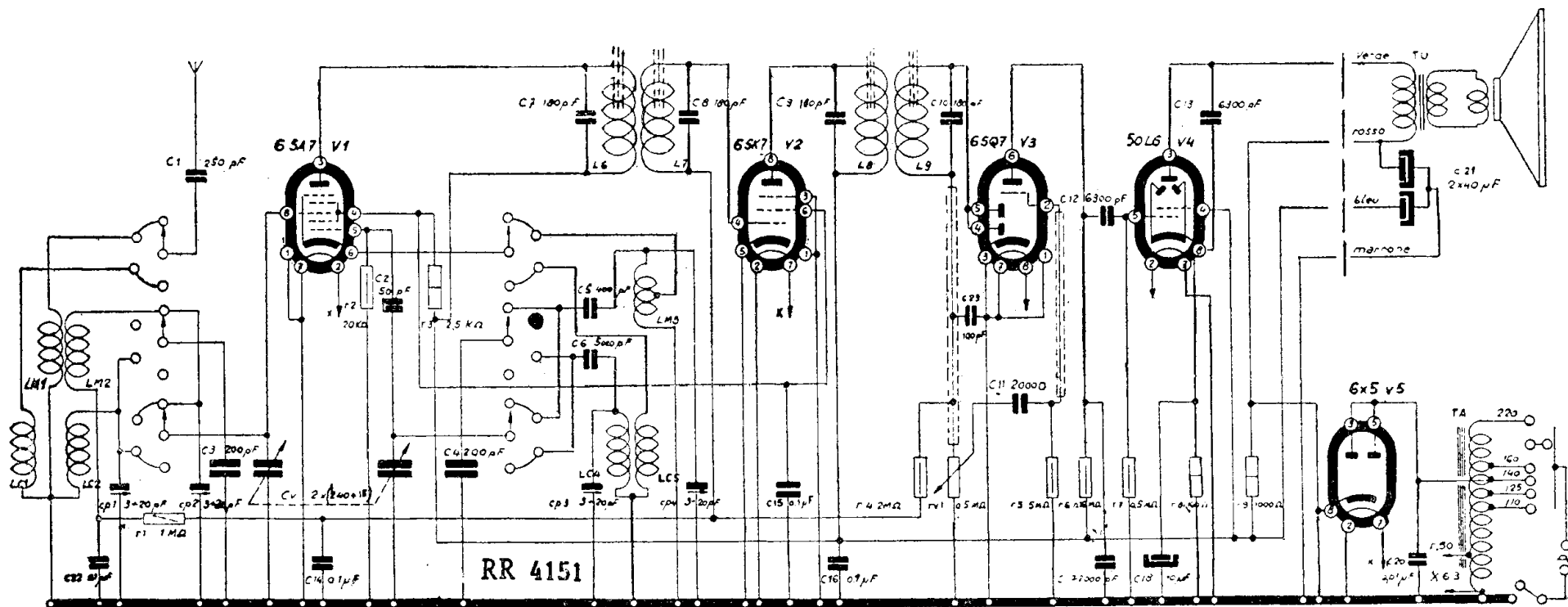
DUCATI - Mod. 4151 - Gamma onde medie divisa, gamme onde corte da 52 a 37 m, e da 40 a 16,5 m. Media frequenza 467 kc. Potenza indistorta d'uscita 1,4 watt. Consumo 47 watt.
